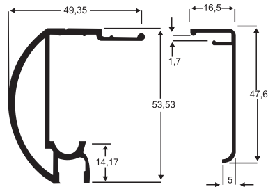
1021-BX 0,717 Kg/m
