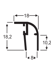
1035-BXC 0,137 Kg/m
