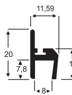
1035-C 0,141 Kg/m
