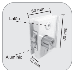
1510M - Mini fechadura c/ um cilindro p/ janela de correr Cerradura pequena p/ ventana de correr (llave de um lado)
