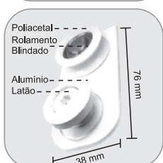
1122M - Mini carrinho simples (1 furo) p/ 1030 (portas até 20 Kg) Carretilla pequena (1 agujero) para perfil 1030 (puertas hasta 20 Kg)
