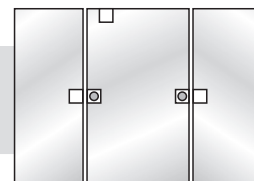
1230 - Dobradiça bucha para basculante 50 x 50 mm Bisagra buje para ventana pivotante 50 x 50 mm
