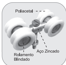
1150 - Roldana quadrupla para trilho 1030 Polea cuadruple para perfil 1030
