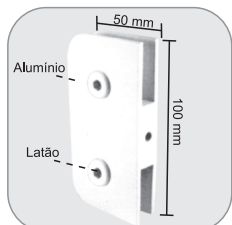
1306 - Suporte para união de 2 vidros Suporte para unión de 2 vidrios
