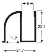
1021-BX 0,717 Kg/m
