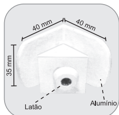
1322 - Suporte de centro c/ núcleo p/ união de 2 vidros a 90° Suporte central con núcleo para unión de 2 vidrios en 90°
