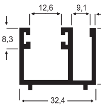
1034-C 0,357 Kg/m
