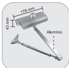
1012S - Mola hidráulica aérea (Cierra puertas) bisagra hidráulica aérea
