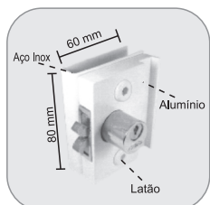
1510MP - Mini fechadura de pressão p/ janela de correr Cerradura pequena de presión para ventana de correr
