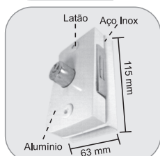
1520XP - Fechadura reforçada de pressão p/ porta de giro Cerradura reforzada de presión para puerta pivotante
