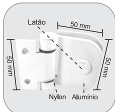
1136 - Dobradiça simples pequena para janela Bisagra lateral pequena para ventana
