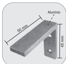
1325 - Suporte para fixação trilho 1030 na parede Suporte para fijación del perfil 1030 en la pared
