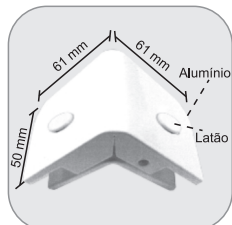
1321 - Suporte piso/teto c/ núcleo p/ união de 2 vidros a 90° Suporte piso y techo con núcleo para unión de 2 vidrios en 90°
