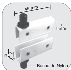
1141 - 2 mini dobradiças pivô de pressão (6 mm) para rack Bisagra pequena con pivote de presión (vidrio 6mm) para mueble
