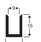
1037-A 0,118 Kg/m
