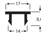
1033 0,097 Kg/m
