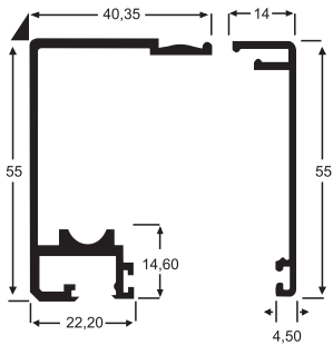
1021-L 0,650 Kg/m
