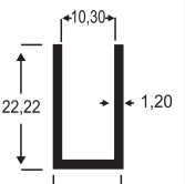
1020 0,181 Kg/m
