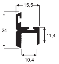
1035-B 0,260 Kg/m
