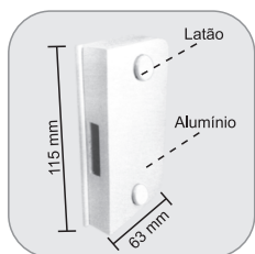
1504X - Contra fechadura para 1520X Contra cerradura para 1520X
