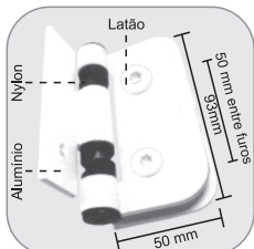
1114 - Dobradiça automática para box Bisagra automática para box (compartimento de ducha)
