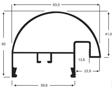
1084 1.098 Kg/m
