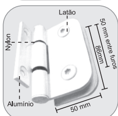
1115 - Dobradiça simples pra box Bisagra simple para box (compartimento de ducha)
