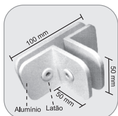
1307 - Suporte sem núcleo para união de 3 vidros em T Suporte "T" sin núcleo para unión de 3 vidrios
