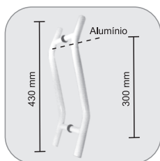
1617 - Puxador tubular em "S" (diâmetro - 25mm) Agarradera en "S" (diámetro 25mm)
