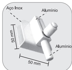
1800C - Trinco de pressão sem núcleo Traba de presión sin núcleo
