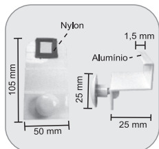
1587V - Conjunto acessório V/V para haste 1587 Acessorios vidro y vidro para brazo 1587
