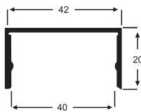
4030-A 0.241 Kg/m
