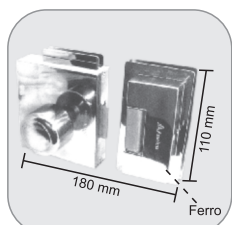
1580 - Fechadura elétrica V/V para recorte Cerradura eléctrica vidrio y vidrio
