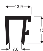
1039-C 0,149 Kg/m
