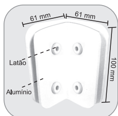
1319 - Suporte para união de 4 vidros a 90° Suporte cuadruple en 90°
