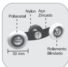
1125D - Roldana dupla com balancim Polea doble con balancín
