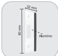
1511AM - Mini testeira para 1510M Chapa pequena en albañilería para cerradura 1510M
