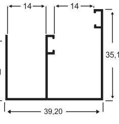
1034-A 0,455 Kg/m
