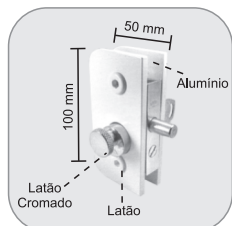
1501 - Fechadura com trinco rolete Cerradura con traba de atornillar
