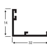
3211 0,245 Kg/m
