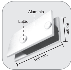
1102M - Mini dobradiça pivotante inferior para 1014 Bisagra pequena inferior para puerta con pivote 1014
