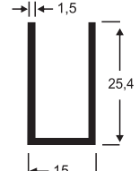
1019 0,210 Kg/m
