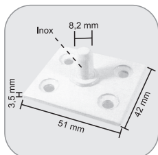
1009G - Max pivô superior para dobradiça 1101G Pivote mayor superior para bisagra 1101G
