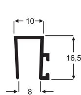
1039 0,166 Kg/m
