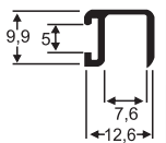
1039-BX 0,094 Kg/m
