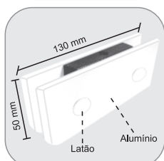
1341 - Suporte de centro com rosca p/ roldana 1150 Suporte central para polea 1150
