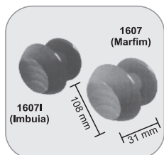
1607I - Puxador de madeira (cor Imbuia) 1607 - Puxador de madeira (cor marfim)
