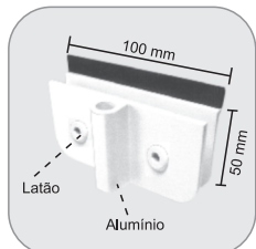
1532 - Contra trinco com aba para 1519 Contra traba con ala para 1519
