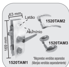
1520TA - Fechadura central p/ maçaneta c/ 2 cilindros Cerradura para manijas
