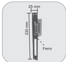
1582 - Fecho eletromagnético V/A Traba electromagnética vidro y albañilería
