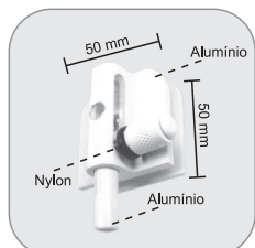
1521L - Trinco com ferrolho lateral Traba de atornillar en la lateral
