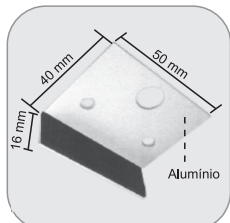
1400 - Batedeira para trinco de basculante Tope para traba de ventana pivotante
