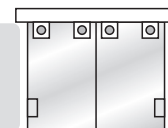
1122M - Mini carrinho simples (1 furo) p/ 1030 (portas até 20 Kg) Carretilla pequena (1 agujero) para perfil 1030 (puertas hasta 20 Kg)
