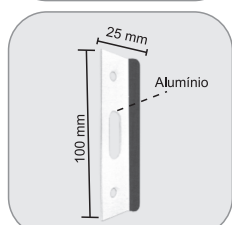
1504A - Batedeira em alvenaria para 1520 e 1550 Tope en albañilería para 1520 y 1550
