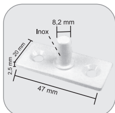
1009 - Pivô para dobradiça 1101, 1230 e 1231 Pivote en acero inoxidable para bisagra 1101, 1230 y 1231
