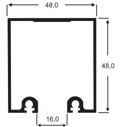
1030-L 0,881 Kg/m
