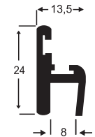
1035 0,242 Kg/m
