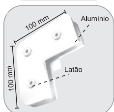
1315 - Suporte sem núcleo com batedeira p/ união de 3 vidros Suporte triple con tope
