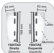
1504TA(D/E) - Contra fechadura s/ maçaneta (vidro fixo) p/ 1520TA Contra cerradura sin manija (vidrio fijo) para 1520TA
