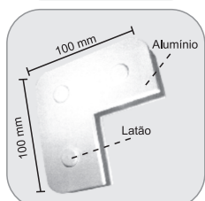
1310 - Suporte sem núcleo para união de 3 vidros Suporte triple
