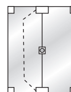
1307 - Suporte sem núcleo para união de 3 vidros em T Suporte "T" sin núcleo para unión de 3 vidrios
