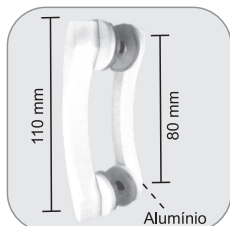
1670D - Puxador duplo p/ portas de correr (80mm entre furos) Agarradera doble para puerta de correr (80mm entre agujeros)
