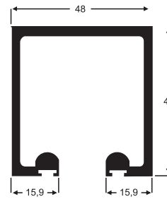
1030 1,209 Kg/m
