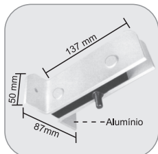
1203 - Suporte de bandeira para dobradiça 1101 Soporte para banderola e bisagra 1101
