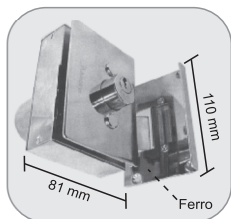
1581 - Fechadura elétrica V/A para recorte Cerradura elétrica vidro y albañilería
