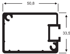
1077 0.813 Kg/m
