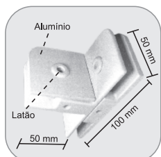
1308 - Suporte com núcleo para união de 3 vidros em T Suporte "T" con núcleo para unión de 3 vidrios
