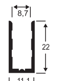
1037-C 0,157 Kg/m
