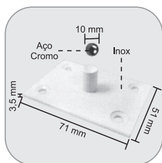
1102G - Max pivô inferior para dobradiça 1102G Pivote mayor inferior para bisagra 1102G
