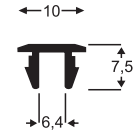
1015 0,097 Kg/m
