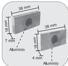
1410 - Contra trinco c/ 4mm auto-adesivo para 1813J 1411 - Contra trinco c/ 7mm auto-adesivo para 1813P Contra traba con 4mm auto-adhesivo para 1813J Contra traba con 7mm auto-adhesivo para 1813P
