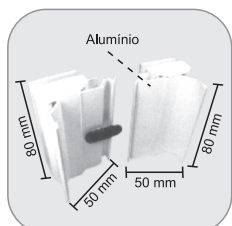
1572 - Fecho central V/V bate-fecha com trava Tope y cierra vidrio y vidrio con traba
