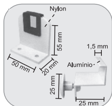
1587A - Conjunto acessório V/A para haste 1587 Acessorios vidro y albañilería para brazo 1587
