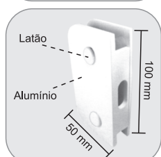
1504 - Contra fechadura para 1520/1550 Contra cerradura para 1520 y 1550
