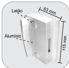
1511X - Contra fechadura para 1510X Contra cerradura para 1510X
