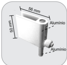
1800AS - Trinco de pressão para janela de correr Traba de presión para ventana de correr
