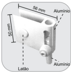
1800 - Trinco para janela de correr Traba para ventana de correr
