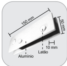
1102 - Dobradiça pivotante inferior para 1014 Bisagra inferior para puerta con pivote 1014
