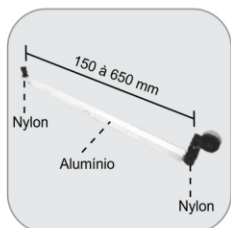
1587 - Haste para MAXIM-AR Brazo para ventana de proyección
