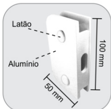
1504 - Contra fechadura para 1520/1550 Contra cerradura para 1520 y 1550
