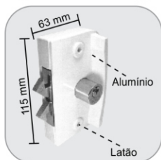
1510X - Fechadura com furação para porta de correr Cerradura para puerta de correr
