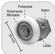
1125E - Roldana para box excêntrica Polea para box excentrica
