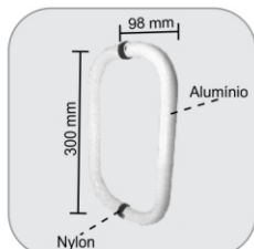
1676 - Puxador tubular com diâmetro de 25 mm (300 mm entre furos) Agarradera con diámetro 25 mm (300 mm entre agujero)
