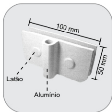
1519A - Contra trinco sem aba para 1519 Contra traba sin ala para 1519
