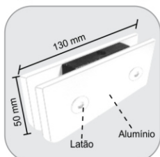
1340 - Suporte de canto com rosca p/ roldana 1150 Suporte de esquina para polea 1150
