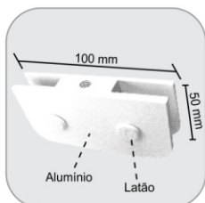
1332 - Suporte central com rosca para 1150S (box) Suporte central para polea 1150S (box)
