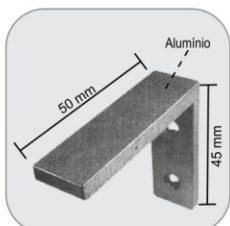
1325 - Suporte para fixação trilho 1030 na parede Suporte para fijación del perfil 1030 en la pared
