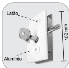
1550 - Fechadura central ou piso com tetra chave Cerradura central y piso con llave tetra
