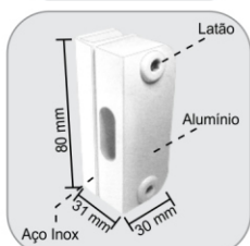
1504P - Contra fechadura de pressão para 1520P Contra cerradura de presión para 1520P
