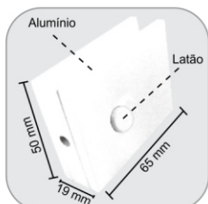
1334 - Grapa para sacada 50 x 65 mm (sem recorte) Grapa para balcón 50 x 65 mm (sin recorte)
