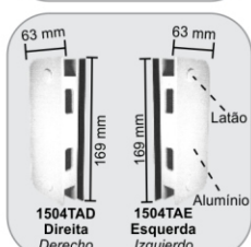
1504TA(D/E) - Contra fechadura s/ maçaneta (vidrio fixo) p/ 1520TA Contra cerradura sin manija (vidrio fijo) para 1520TA
