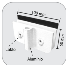
1532 - Contra trinco com aba para 1519 Contra traba con ala para 1519
