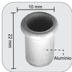
1200 - Capuchinho para trinco e fechadura Contra traba y cerradura de piso
