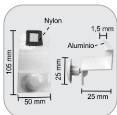
1587V - Conjunto acessório V/V para haste 1587 Acessorios vidrio y vidrio para brazo 1587
