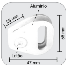
1671MD - Mini puxador duplo com transpasse para portas e janelas com um furo
