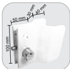
1520PX - Fechadura 1520 c/ puxador embutido Cerradura 1520 con agarradera embutida
