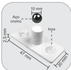
1014 - Pivô inferior para dobradiça 1102 Pivote inferior para bisagra 1102
