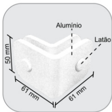
1320 - Suporte central s/ núcleo p/ união de 2 vidros a 90° Suporte central sin núcleo para unión de 2 vidrios en 90°
