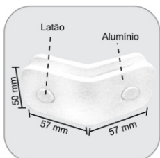
1321A - Suporte central s/ núcleo p/ união de 2 vidros a 135° Suporte central sin núcleo para unión de 2 vidrios en 135°
