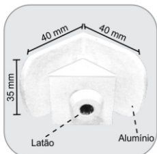
1322 - Suporte de centro c/ núcleo p/ união de 2 vidros a 90° Suporte central con núcleo para unión de 2 vidrios en 90°
