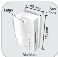
1511XP - Contra fechadura de pressão para 1510XP Contra cerradura de presión para 1510XP
