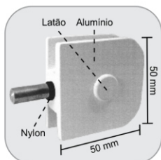
1123 - Dobradiça para basculante 50 x 50 mm Bisagra vidrio y vidrio para ventana pivotante
