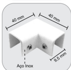
1350 - Suporte superior p/ box a 90° (sem recorte) Suporte superior para box en 90° (sin recorte)
