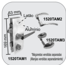
1520TA - Fechadura central p/ maçaneta c/ 2 cilindros Cerradura para manijas
