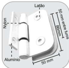
1115 - Dobradiça simples pra box Bisagra simple para box (compartimiento de ducha)
