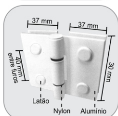
1131 - Dobradiça maxin-ar V/V 40 mm entre furos Bisagra vidrio y vidrio p/ ventana de preyección (40 mm entre agujeros)
