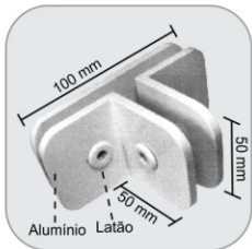
1307 - Suporte sem núcleo para união de 3 vidros em T Soporte "T" sin núcleo para unión de 3 vidrios
