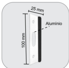
1504A - Batedeira em alvenaria para 1520 e 1550 Tope en albañilería para 1520 y 1550
