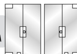
1504TAM(D/E) - Contra fechadura p/ maçaneta (2 portas) p/ 1520TA Contra cerradura con manijas (2 puertas) para 1520TA
