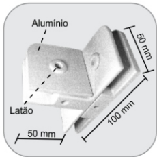
1308 - Suporte com núcleo para união de 3 vidros em T Soporte "T" con núcleo para unión de 3 vidrios
