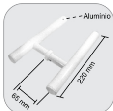
1696 - Puxador tubular tipo H (diâmetro 25 mm) Agarradera "H" (Diámetro 25 mm)
