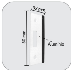
1511AM - Mini testeira para 1510M Chapa pequena en albañilería para cerradura 1510M
