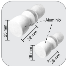
1629 - Puxador para box (25mm) 1630 - Puxador para box (19mm)
