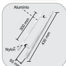
1679 - Puxador tubular reto 25 mm (300 mm entre furos) 1679A - Puxador tubular reto 25 mm (especial)
