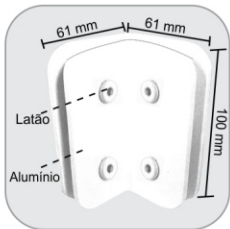
1319 - Suporte para união de 4 vidros a 90° Soporte cuadruple en 90°
