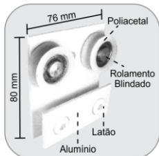
1122 - Carrinho duplo para 1030 (portas até 80 Kg) Carretilla doble para perfil 1030 (puerta hasta 80Kg)
