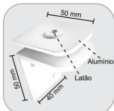
1333 - Suporte para prateleiras Suporte para repisas
