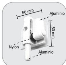
1521L - Trinco com ferrolho lateral Traba de atornillar en la lateral
