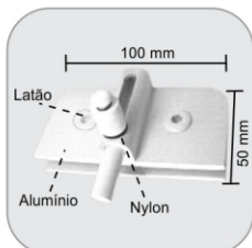
1519 - Trinco inferior sem núcleo 50x100 mm Traba inferior sin núcleo 50x100 mm
