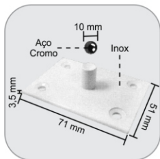
1014G - Max pivô inferior para dobradiça 1102G Pivote mayor inferior para bisagra 1102G
