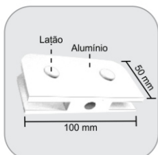
1231 - Dobradiça bucha para basculante 50 x 100 mm Bisagra buje para ventana pivotante 50 x 100 mm
