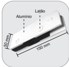
1103 - Dobradiça inferior para mola de piso Bisagra inferior para cierra puertas 1012
