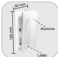
1511 - Contra fechadura com aba de proteção para 1510 Contra cerradura con ala para 1510
