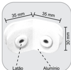
1335 - Suporte para união de 2 vidros a 135° Suporte para unión de 2 vidrios en 135°
