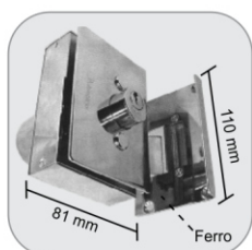
1581 - Fechadura elétrica V/A para recorte Cerradura eléctrica vidrio y albañilería
