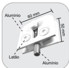
1813J - Trinco p/ janela de correr que permite transpasse Traba para ventana de correr (permite traspasar)
