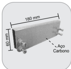
1906P - Suporte p/ mola aérea (porta) (dispensa recorte) Soporte para bisagra hidráulica aérea (puerta)
