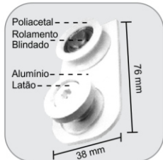
1122M - Mini carrinho simples (1 furo) p/ 1030 (portas até 20 Kg) Carretilla pequeña (1 agujero) para perfil 1030 (puertas hasta 20 Kg)
