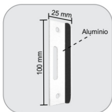
1504AF - Batedeira em alvenaria para 1520BF Tope en albañilería para 1520BF
