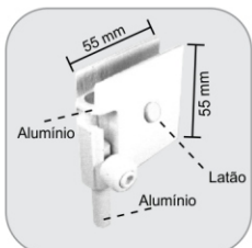
1810E - Trinco esquerdo para janela de correr Traba izquierda para ventana de correr
