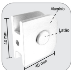
1326 - Mini suporte para fixação 40 x 40 mm Suporte pequeño central 40 x 40 mm
