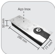
1012 - Mola Hidráulica de piso (Cierra puertas) bisagra hidráulica de piso
