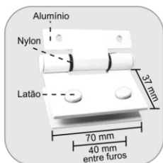
1132 - Dobradiça maxim-ar V/A 40 mm entre furos Bisagra V/A para ventana de proyección (40 mm entre agujeros)
