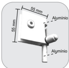
1810D - Trinco direito para janela de correr Traba derecha para ventana de correr
