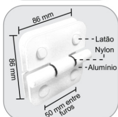
1134 - Dobradiça maxim-ar V/V 50 mm entre furos Bisagra V/V para ventana de proyección (50 mm entre agujeros)
