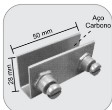
1906 - Suporte p/ mola aérea (bandeira) (dispensa recorte) Soporte para bisagra hidráulica aérea (banderola)
