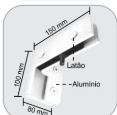
1209E - Facão esquerdo à 90° para 1101 Soporte "L" izquierdo en 90° para bisagra 1101 y banderola
