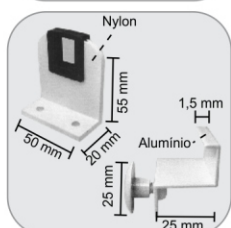
1587A - Conjunto acessório V/A para haste 1587 Acessorios vidrio y albañilería para brazo 1587
