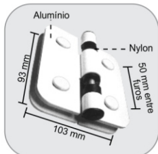
1114D - Dobradiça dupla automática direita Bisagra automática para box vidro y vidrio derecha
