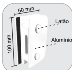
1531BF - Contra fechadura com batente para 1520BF Contra cerradura con tope para 1520BF
