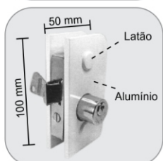
1520BF - Fechadura de centro bate-fecha Cerradura con tope y cierra
