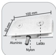
1130 - Dobradiça p/ basculante c/ pino 50 x 100 mm Bisagra vidrio y vidrio para ventana pivotante
