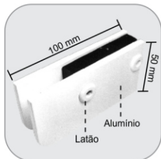
1101M - Mini dobradiça pivotante superior para 1014 Bisagra pequeña superior para puerta con pivote 1014
