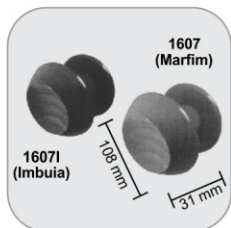
1607I - Puxador de madeira (cor Imbuía) 1607 - Puxador de madeira (cor marfim)
