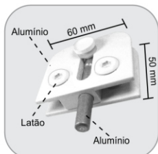
1813P - Trinco p/ porta de correr que permite transpasse Traba para puerta de correr (permite traspasar)
