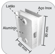
1511MP - Mini contra fechadura de correr de pressão p/ 1510MP Contra cerradura pequena de presión para 1510MP
