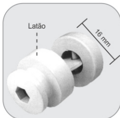
1001L - Botão de correção lâmina com engate Botón de corrección lámina con enganche
