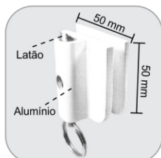
1523 - Trinco central para basculante Traba para ventana pivotante
