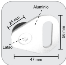
1671M - Mini puxador para transpasse portas e janelas com um furo
