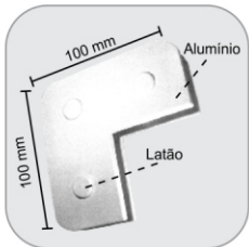
1310 - Suporte sem núcleo para união de 3 vidros Soporte triple
