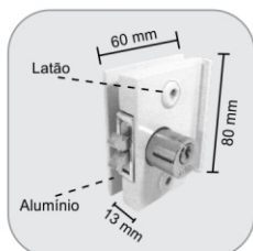
1510M - Mini fechadura c/ um cilindro p/ janela de correr Cerradura pequeña p/ ventana de correr (llave de um lado)
