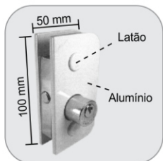
1520 - Fechadura central ou piso com 2 cilindros Cerradura central y piso para puerta pivotante
