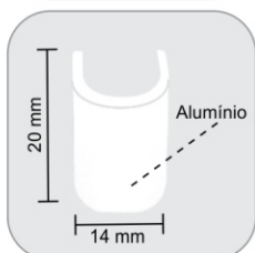
1408 - Contra trinco para 1519 e 1521 Contra traba 1519 y 1521
