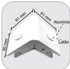
1321 - Suporte piso/teto c/ núcleo p/ união de 2 vidros a 90° Suporte piso y techo con núcleo para unión de 2 vidrios en 90°
