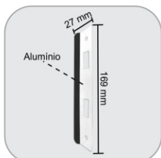
1504ATE - Batedeira em alvenaria p/ 1520TA esquerda (vista externa) Tope en albañilería p/ 1520TA izquierdo (vista externa)
