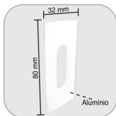
1672 - Puxador auto-adesivo para transpasse Agarradera auto adhesivo (permite traspasar)
