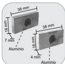
1410 - Contra trinco c/ 4mm auto-adesivo para 1813J 1411 - Contra trinco c/ 7mm auto-adesivo para 1813P
