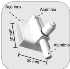
1800C - Trinco de pressão sem núcleo Traba de presión sin núcleo
