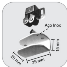
1704 - Fixador de pressão para portas de extintores Fijador de presión para puerta de aparato contra incendios
