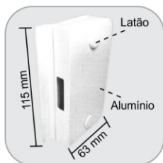
1531X - Contra Fechadura para 1520X Contra cerradura para 1520X
