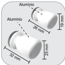
1650 - Puxador para janela de correr (25mm) 1651 - Puxador para janela de correr (19mm)
