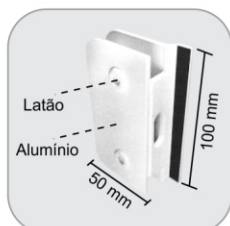
1531 - Contra fechadura com batente p/ 1520 e 1550 Contra cerradura con tope para 1520 y 1550
