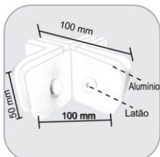
1323 - Suporte p/ união de 4 vidros perpendiculares Suporte para unión de 4 vidrios perpendiculares
