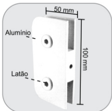
1306 - Suporte para união de 2 vidros Soporte para unión de 2 vidrios
