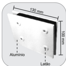
1101G - Max dobradiça superior para 1009G Bisagra mayor para puerta con pivote 1009G
