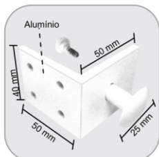
1336 - Cantoneira completa p/ sistema "só vidro" c/ 1006 Esquinera completa para sistema "sólo vidrio" con 1006
