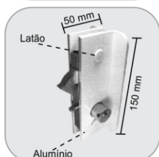
1510 - Fechadura bico-de-papagaio com pino e trava Cerradura para puerta de correr con perno y traba
