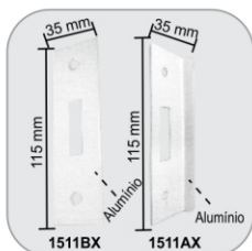
1511BX - Testeira para 1510X e 1520X no piso 1511AX - Testeira para 1510X
