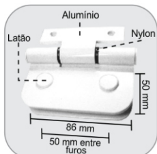
1133 - Dobradiça maxim-ar V/A 50 mm entre furos Bisagra V/A para ventana de protección (50 mm entre agujeros)
