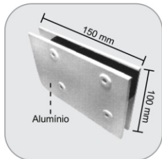
1102G - Max dobradiça pivotante inferior para 1014G Bisagra mayor inferior para puerta con pivote 1014G
