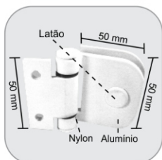
1136 - Dobradiça simples pequena para janela Bisagra lateral pequena para ventana
