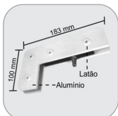
1209 - Facão simples para bandeira e fixo para 1101 (Pistola) soporte "L" para bisagra 1101 y banderola
