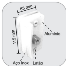
1510XP - Fechadura de pressão para porta de correr Cerradura de presión para puerta de correr
