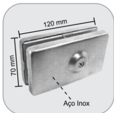
1500 - Fechadura de encaixar p/ porta pivotante Cerradura de encaje para puerta pivotante
