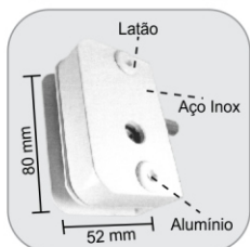
1520P - Fechadura de pressão com tetra chave Cerradura de presión con llave tetra
