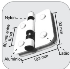
1114E - Dobradiça dupla automática esquerda Bisagra automática para box vidro y vidrio izquierda
