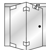
1341 - Suporte de centro com rosca p/ roldana 1150 Suporte central para polea 1150
