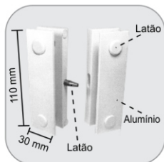
1710 - Conjunto mão-de-amigo p/ portas de correr com 1030 Sistema de trabar y tirar para puertas de correr con perfil 1030
