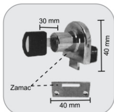
1913P - Fechadura de pressão com lingueta para rack Cerradura de presión para mueble
