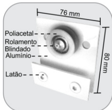
1122S - Carrinho simples (2 furos) p/ 1030 (portas até 30Kg) Carretilla (2 agujeros) para perfil 1030 (puertas hasta 30 Kg)
