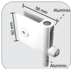
1800A - Trinco para janela de correr Traba para ventana de correr
