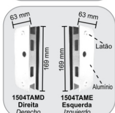
1504TAM(D/E) - Contra fechadura p/ maçaneta (2 portas) p/ 1520TA Contra cerradura con manijas (2 puertas) para 1520TA
