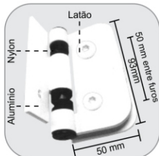
1114 - Dobradiça automática para box Bisagra automática para box (compartimiento de ducha)
