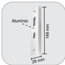
1511A - Testeira de parede para 1510 Chapa em albañilería para cerradura 1510
