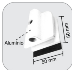
1525 - Contra trinco com aba p/ 1521 e 1523 Contra traba con ala para 1521 y 1523
