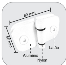
1137 - Dobradiça dupla pequena para janela Bisagra lateral pequena vidro y vidrio para ventana
