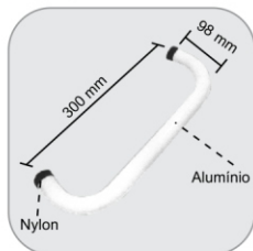
1680 - Puxador tubular p/ porta sanfonada (300 mm entre furos)
