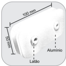
1305 - Suporte central sem núcleo Soporte central sin núcleo
