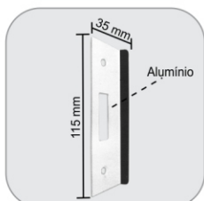
1504AX - Batedeira em alvenaria p/ 1520X (c/ borracha) Tope en albañilería para 1520X
